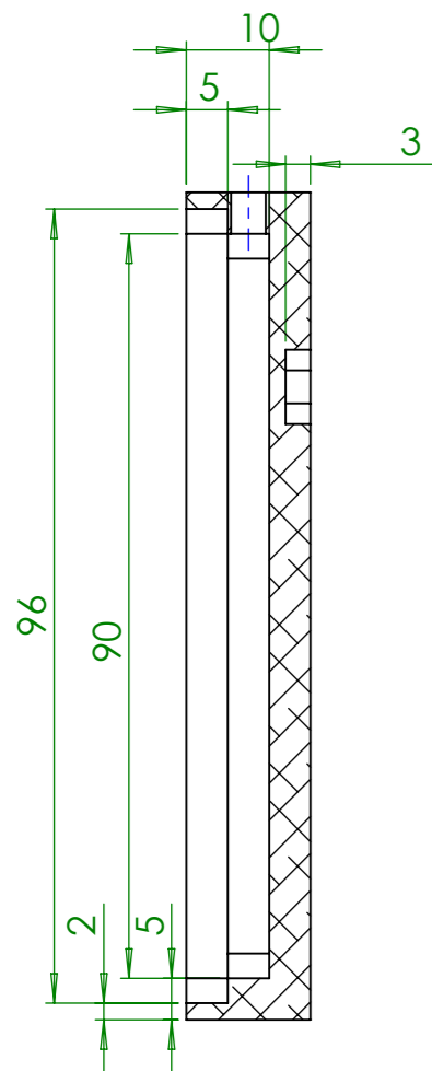
SECTION A-A
